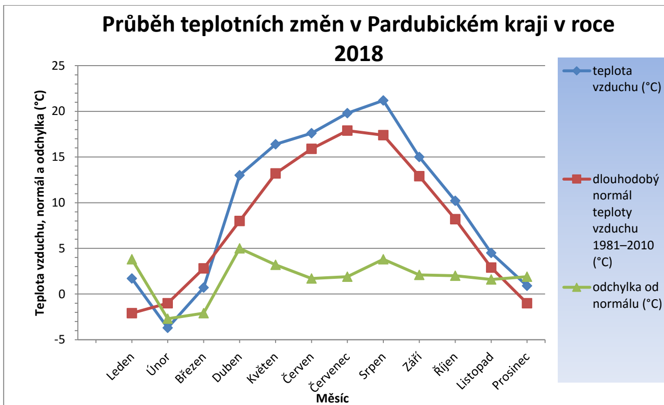
Obrázek 41: Grafické znázornění teploty vzduchu a porovnání s dlouhodobým normálem teplot (°C) v období 1981–2010 v Pardubickém kraji (2018); hodnoty převzaty z http://portal.chmi.cz
