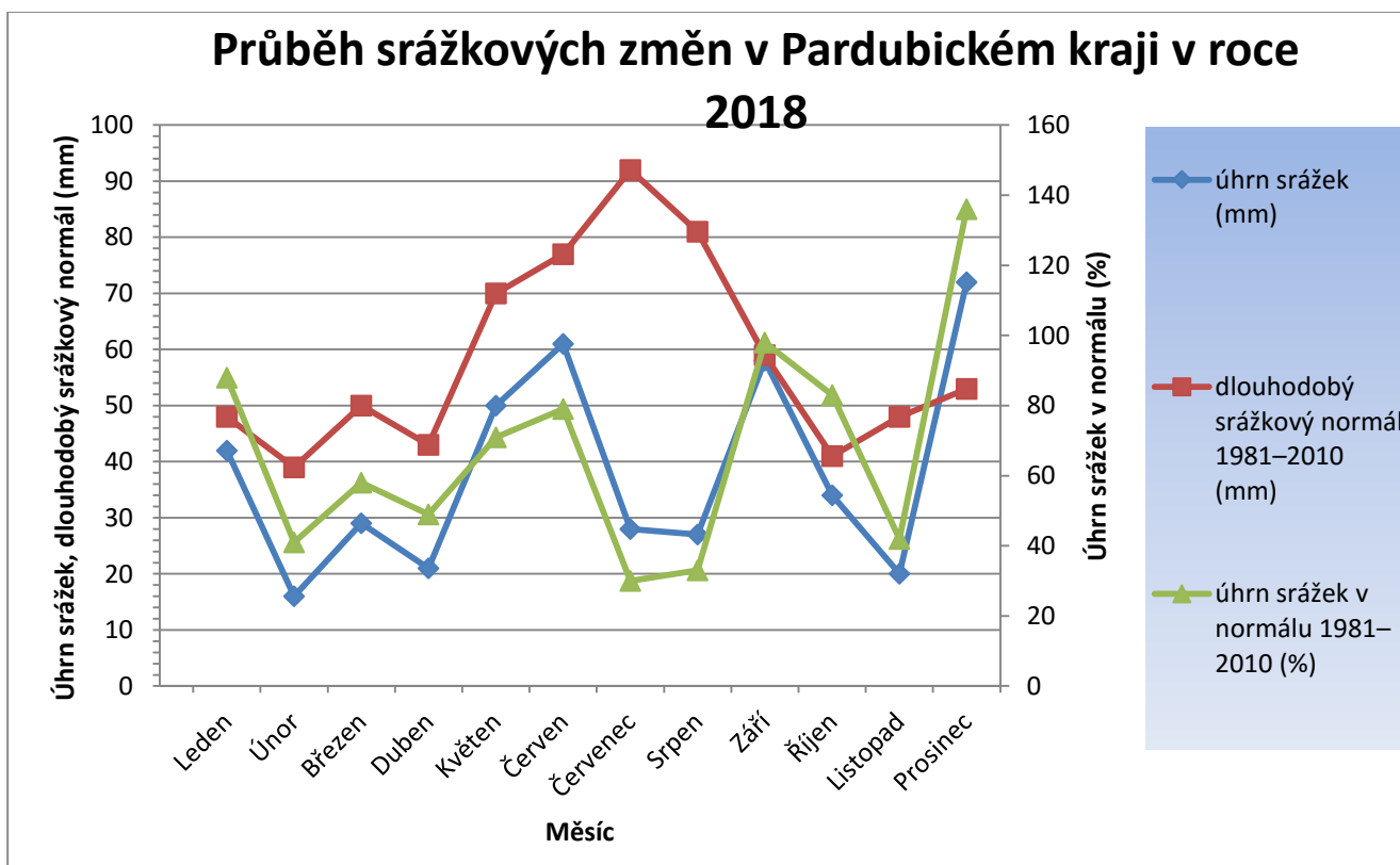
Obrázek 42: Grafické znázornění úhrnu srážek a porovnání s dlouhodobým srážkovým (mm) normálem v období 1981–2010 v Pardubickém kraji (2018); hodnoty převzaty z http://portal.chmi.cz
