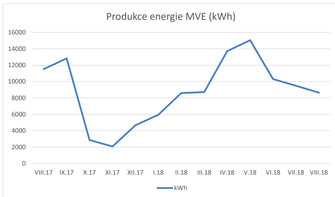
Obrázek 2: Graf znázorňující produkci elektrické energie malou vodní elektrárnou v období 8. 2017 až 8. 2018
