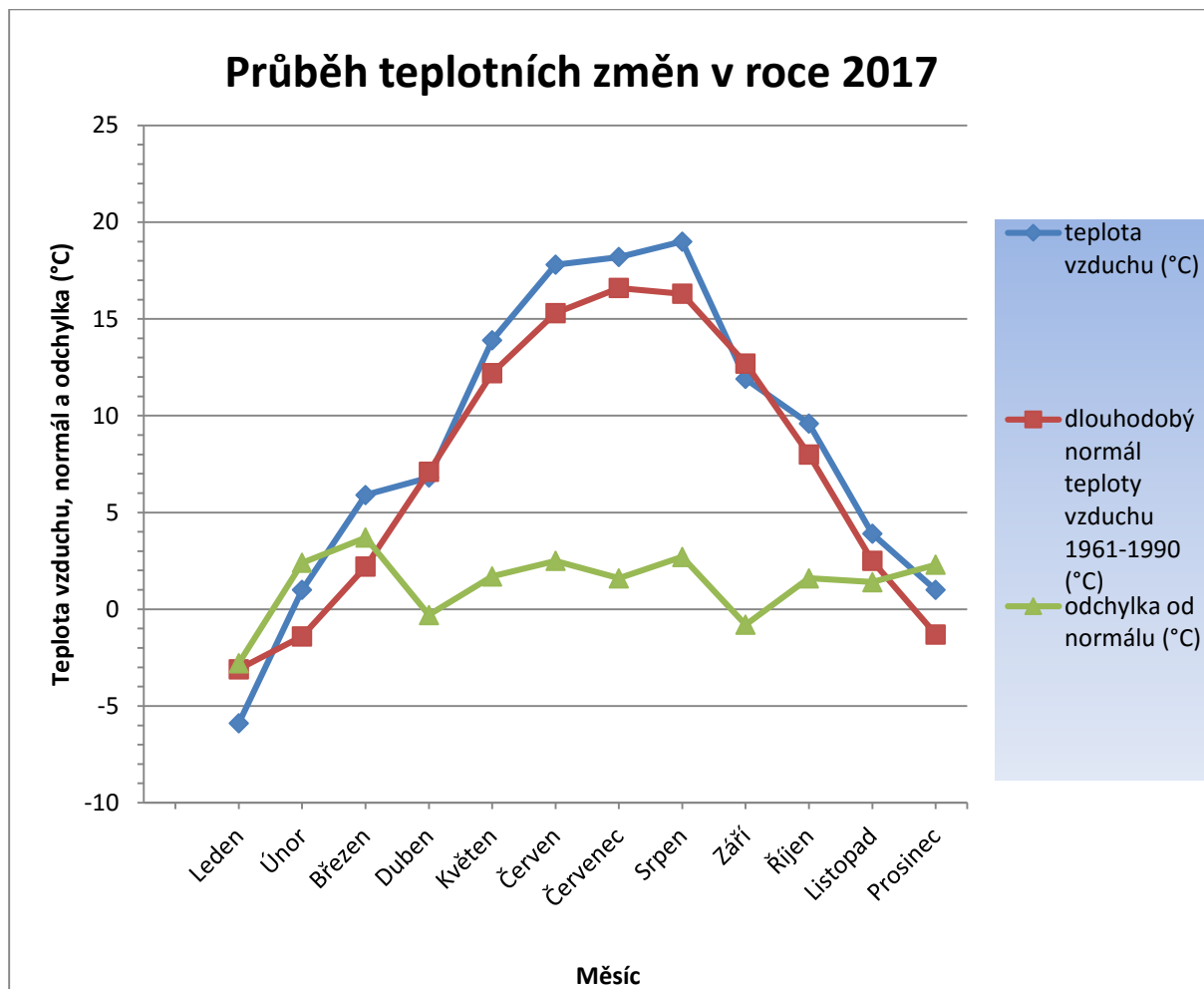
Obrázek 55: Grafické znázornění teploty vzduchu a porovnání s dlouhodobým normálem teplot (°C) 1961-1990 v Pardubickém kraji (2017); hodnoty převzaty z http://portal.chmi.cz/portal/dt?menu=JSPTabContainer/P4_Historicka_data/P4_1_Pocasi/P4_1_1_Zakl_Info
