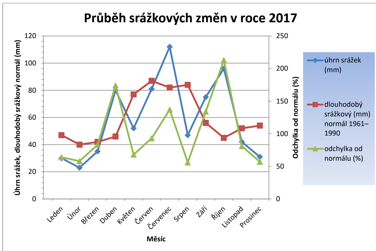
Obrázek 54: Grafické znázornění úhrnu srážek a porovnání s dlouhodobým srážkovým (mm) normálem 1961–1990 v Pardubickém kraji (2017); hodnoty převzaty z http://portal.chmi.cz/portal/dt?menu=JSPTabContainer/P4_Historicka_data/P4_1_Pocasi/P4_1_1_Zakl_Info
