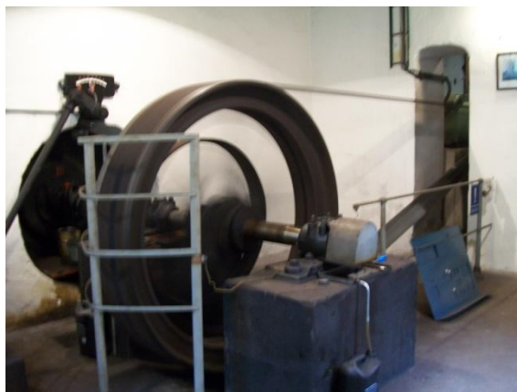
Obrázek 3: Pohled na část strojího zařízení malé vodní elektrárny výrovského mlýna (Stav k 20. 7. 2012)
