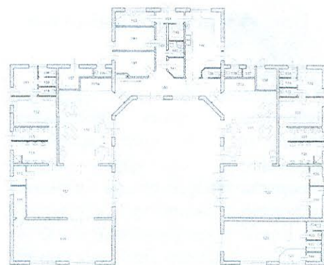
Půdorys nové mateřské školky
